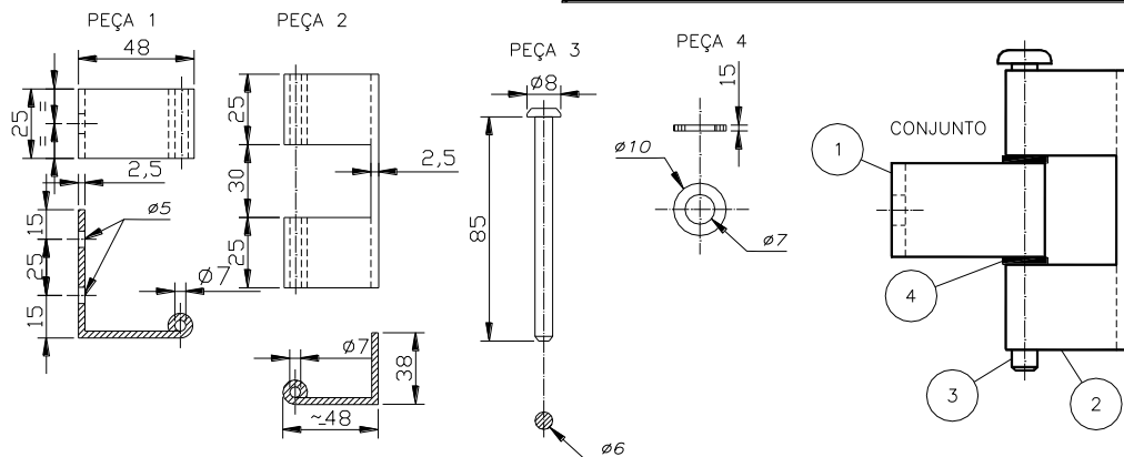
DETALHE B (DOBRADIÇA)
